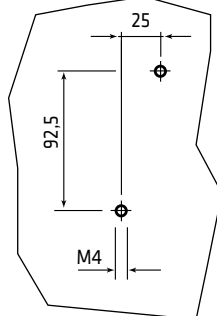
Задняя стенка Винтовое крепление Серия SE63-SE80-SE100
